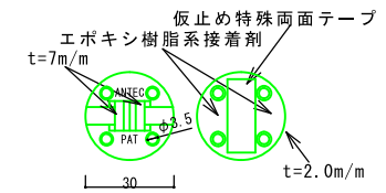
特殊取付具ピット詳細図 (S=1/2)
