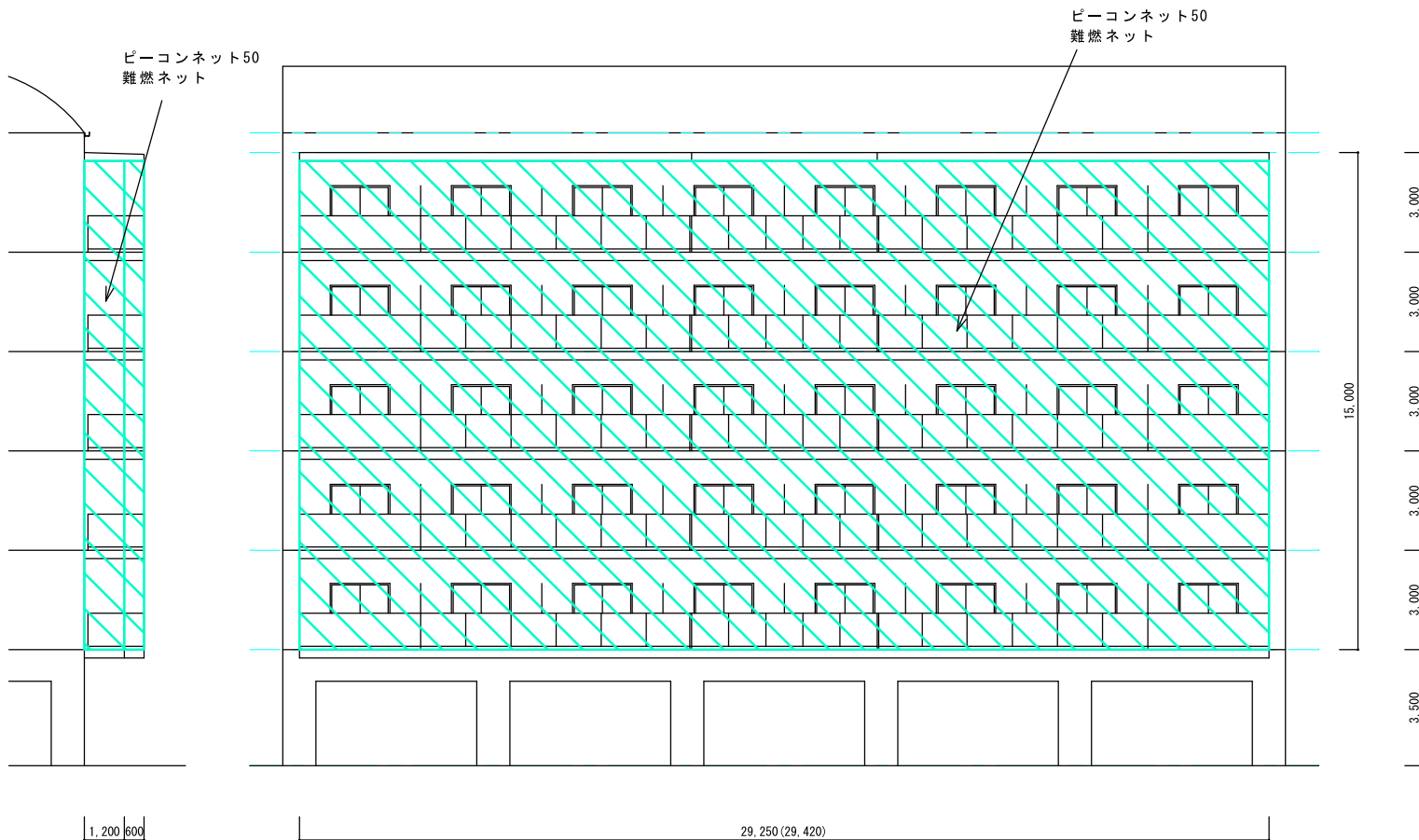
東面立面図 (S=1/150)
